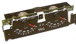
CÓDIGO: 777.120.335F004 DESCRIÇÃO: MANÔMETROS, PLACA DE CIRCUITO, MOSTRADOR E PONTEIROS - AZUL, VERSÃO DE TETO
