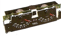
CÓDIGO: 777.120.335F006 DESCRIÇÃO: MANÔMETROS, PLACA DE CIRCUITO, MOSTRADOR E PONTEIROS - ÂMBAR, VERSÃO DE TETO
