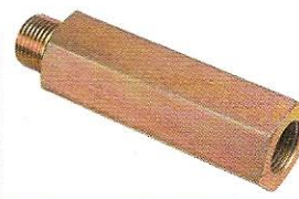
CÓDIGO: 777.120.520F DESCRIÇÃO: EXTENSÃO 85 mm
